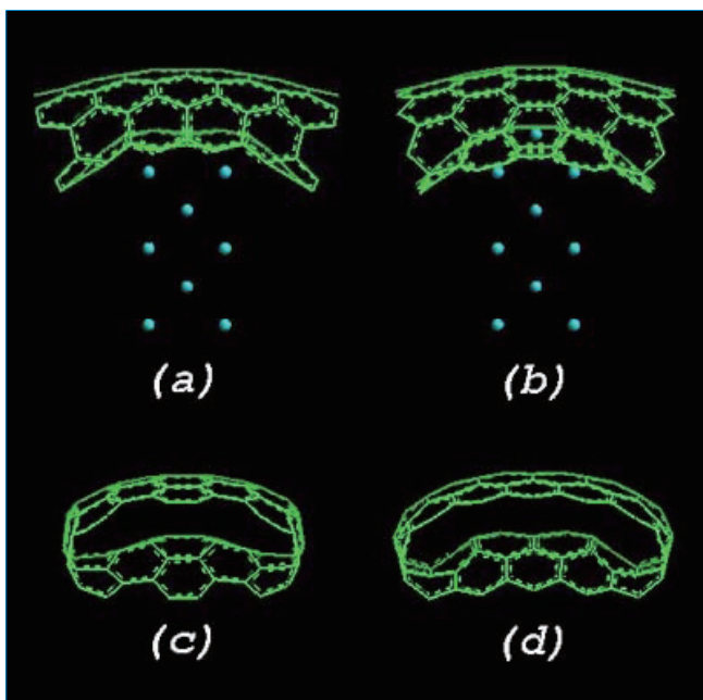
図1 DMol 3 で緩和させた(a): (6, 6)アームチェアー(1 3 2炭素原子)、および(b): (1 2, 0)ジグザグ型(1 4 4炭素原子)のLiチップで変形させたクラスター。変形角はどちらも25°。(c)、(d)はナノチューブの軸方向からの図。sp 3 配位が無いことを明確に示している。チューブの他の部分は古典的力場計算で表現されているが、ここでは分かり易くするために表示していない。
