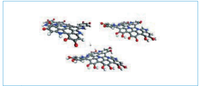
図1 DFTで最適化した六量体のDHIメラニン構造(a)酸化型, (b)半還元型, (c)全還元型。炭素原子はグレー、酸素原子は赤、窒素原子は青、水素原子は白で示されています。
