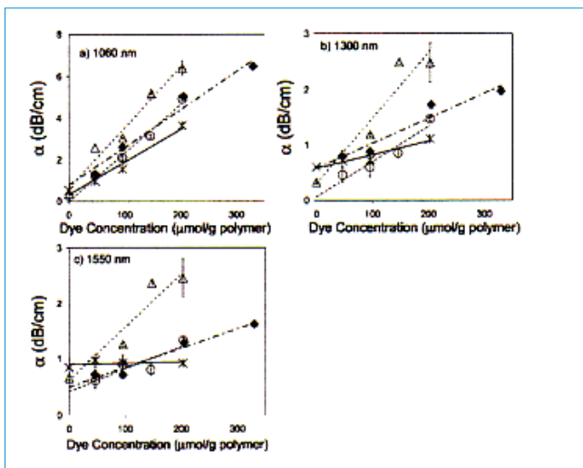
図3: 図2の4E6m/Bisphenol A polycarbonate系についてのPDS吸収損失を、3つの異なる波長で測定したもの
